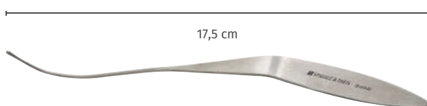
Nasensonde, s-förmig gebogen, biegsam, 17,5 cm Nasal probe, s-shaped, bendable, 17.5 cm
